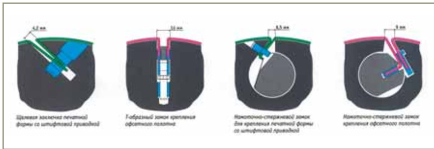
Система крепления формных и офсетных цилиндров
